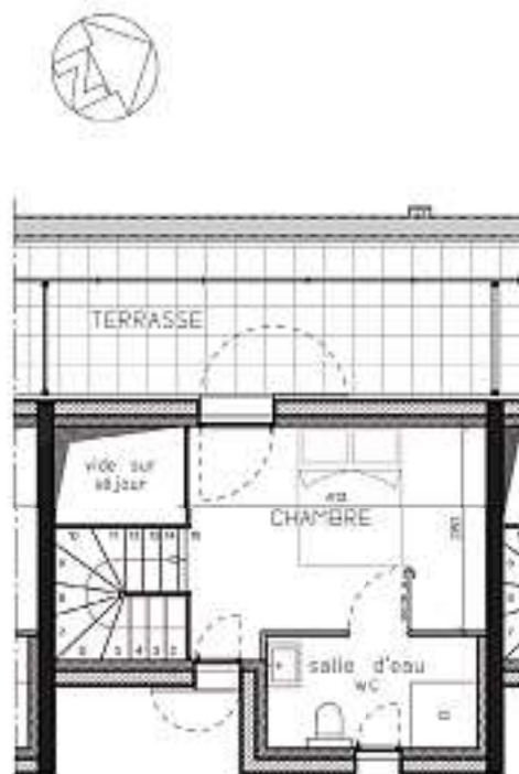
plan étage
