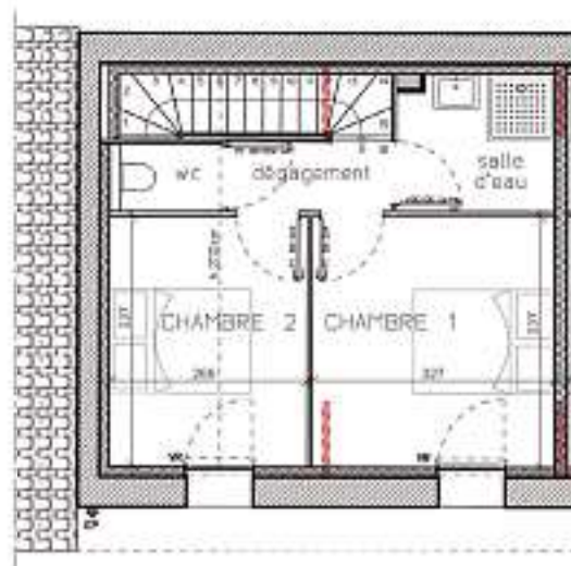
plan étage
