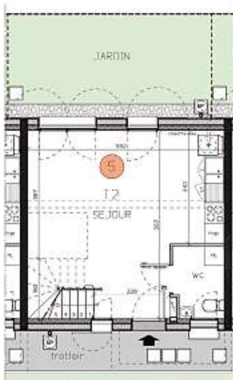
plan rez-de-chaussée
